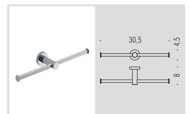
W4990 Porta rotolo doppio Double Paper holder
