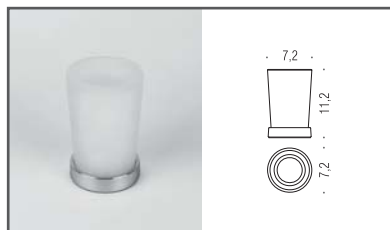
B8041 Porta bicchiere d'appoggio Standing glass holder
